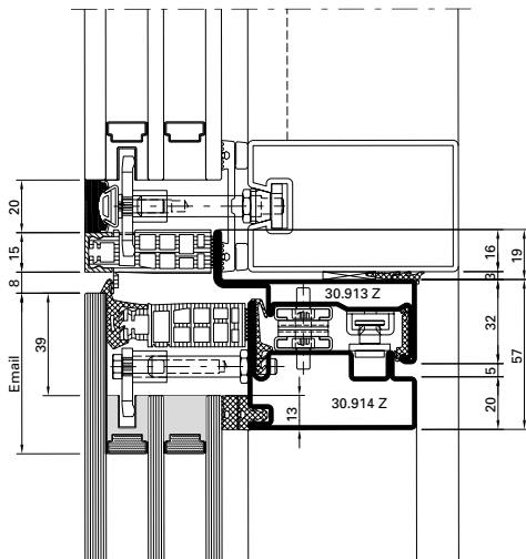
Parallelausstellfenster VISS SG 50 mm Fenster ohne mechanische Sicherung der Aussenscheibe
