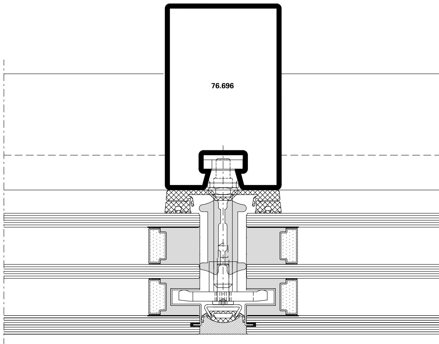
VISS SG HI Détail de la montante Largeur de face 50 mm
