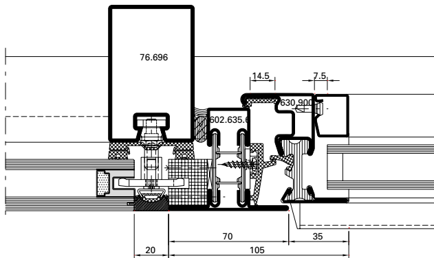
Einsatzelement Fenster Élément de remplissage fenêtre Infill element window
