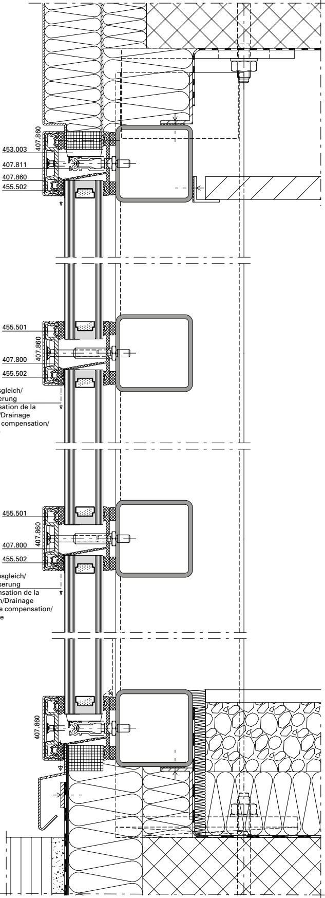
B-B (Schraubbolzen/Goujon à visser/Screw bolt)
