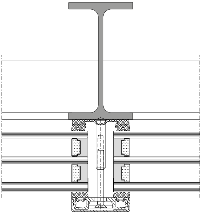
VISS Basic Semi SG Ansichtsbreite 50 mm Schweissbolzen
