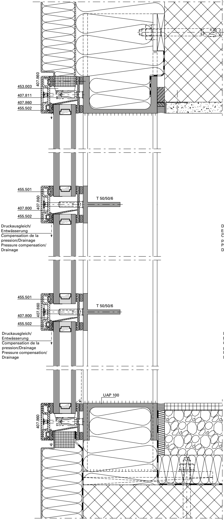
B-B (Schweissbolzen/Goujon à souder/Welding stud)
