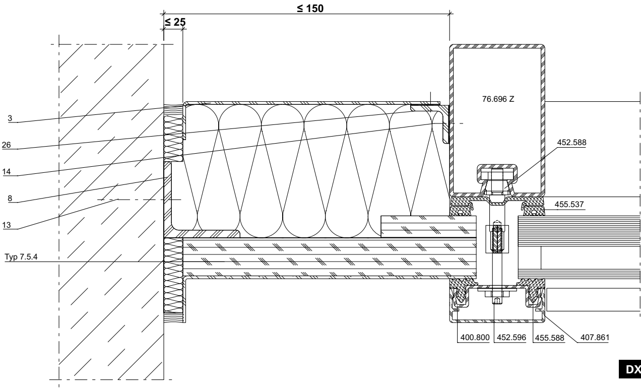
Wandanschluss
