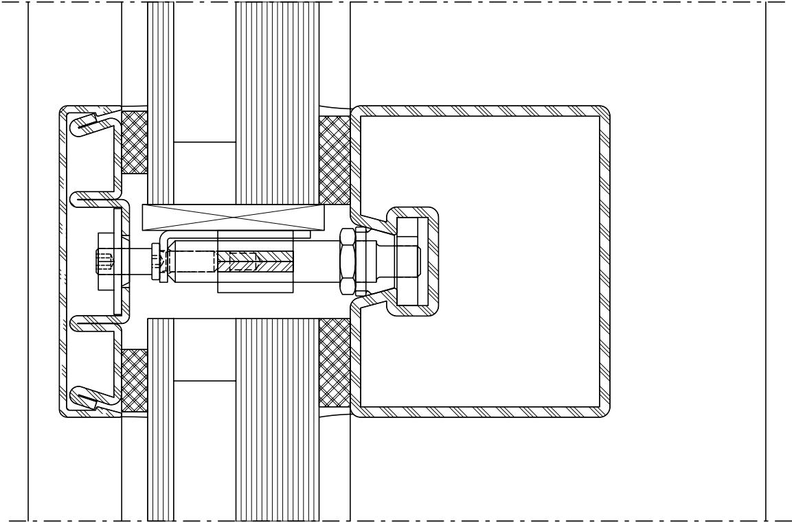
Riegel-Detail Ansichtsbreite 60 mm Trennwandlösung (nur Innenanwendung)
