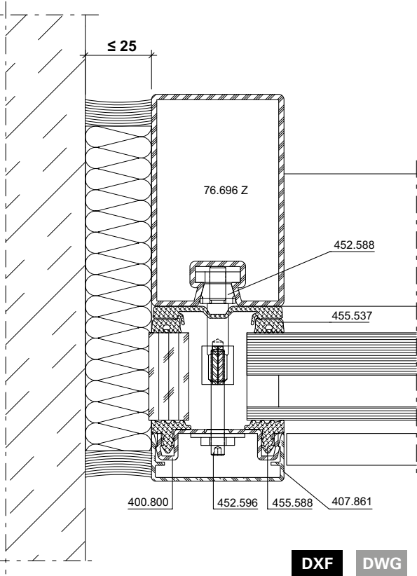
Wandanschluss
