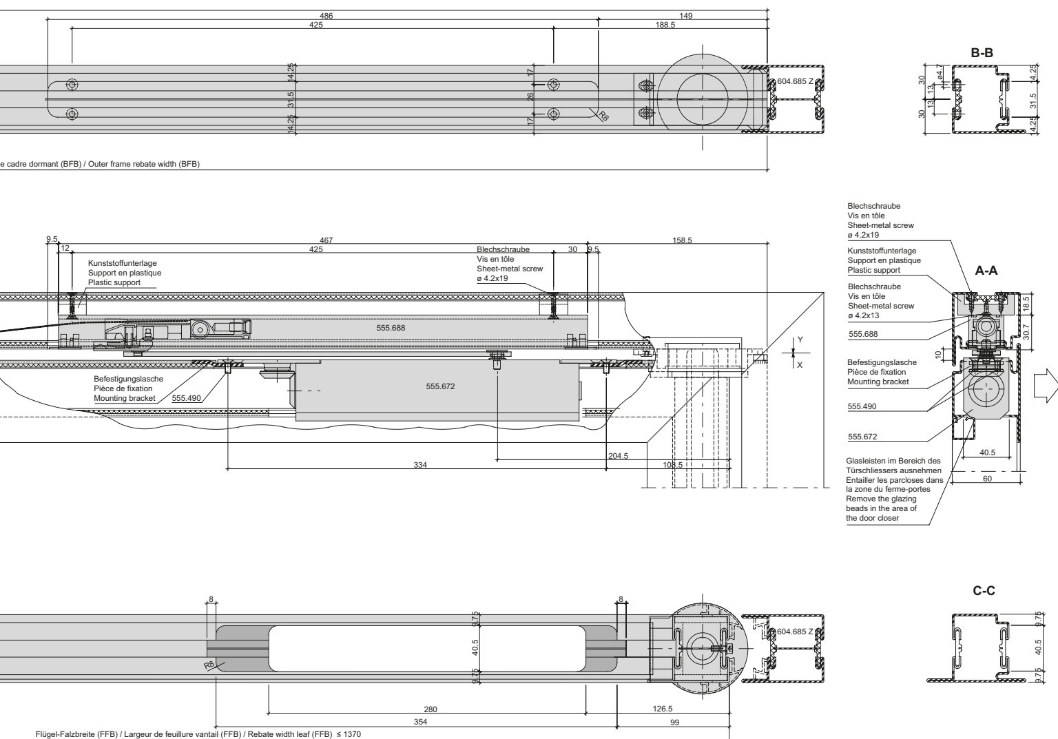
Abbildung: Gleitschiene 550.385
