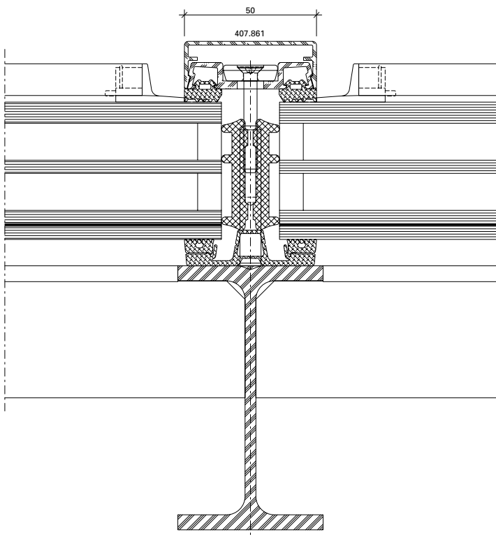
Détail du chevron HI Largeur de face 50 mm Goujon à souder
