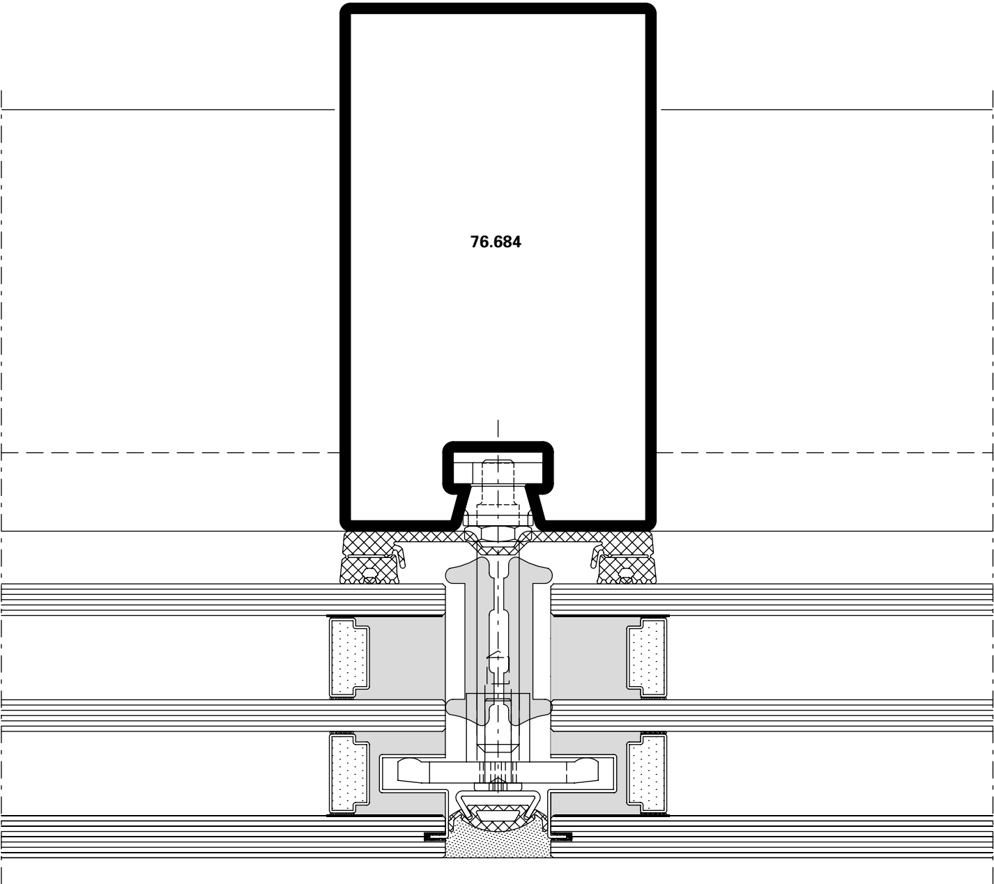
VISS SG HI Pfoften-Detail Ansichtsbreite 60 mm
