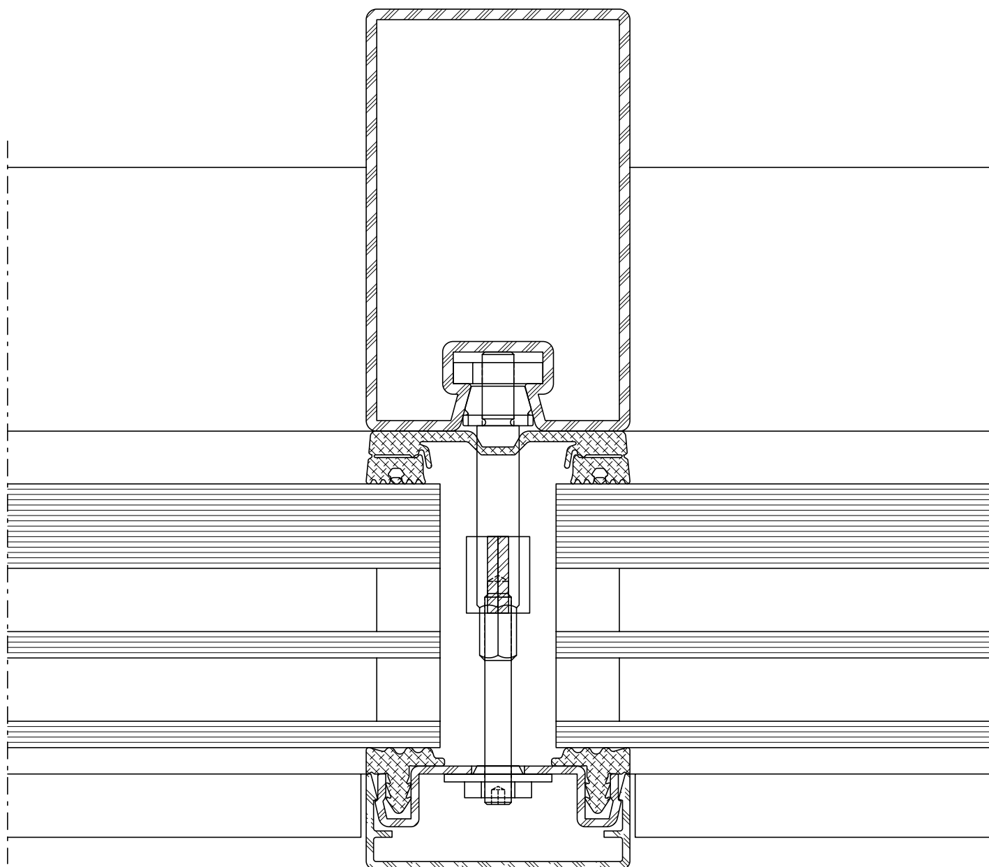
Détail du montant Largeur de face 50 mm
