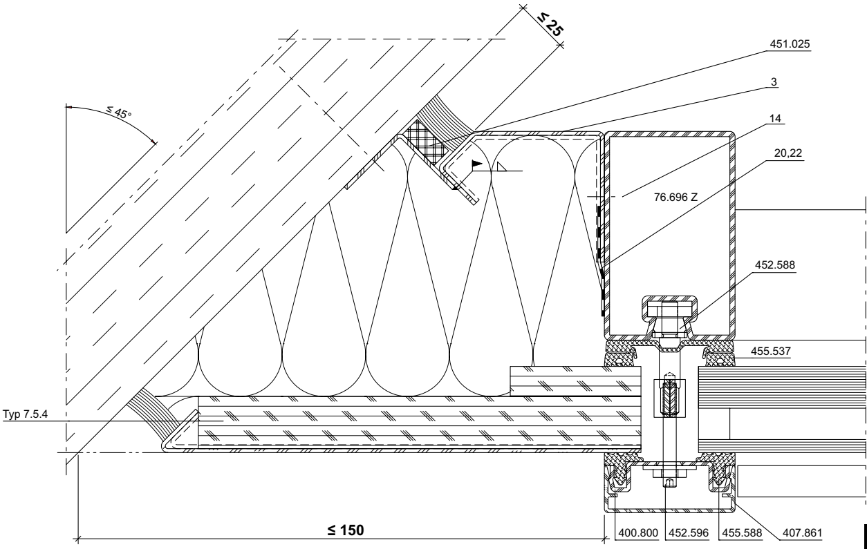
Wandanschluss
